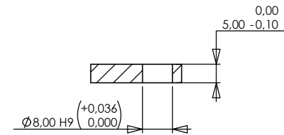
SEZIONE B-B (section B-B)
