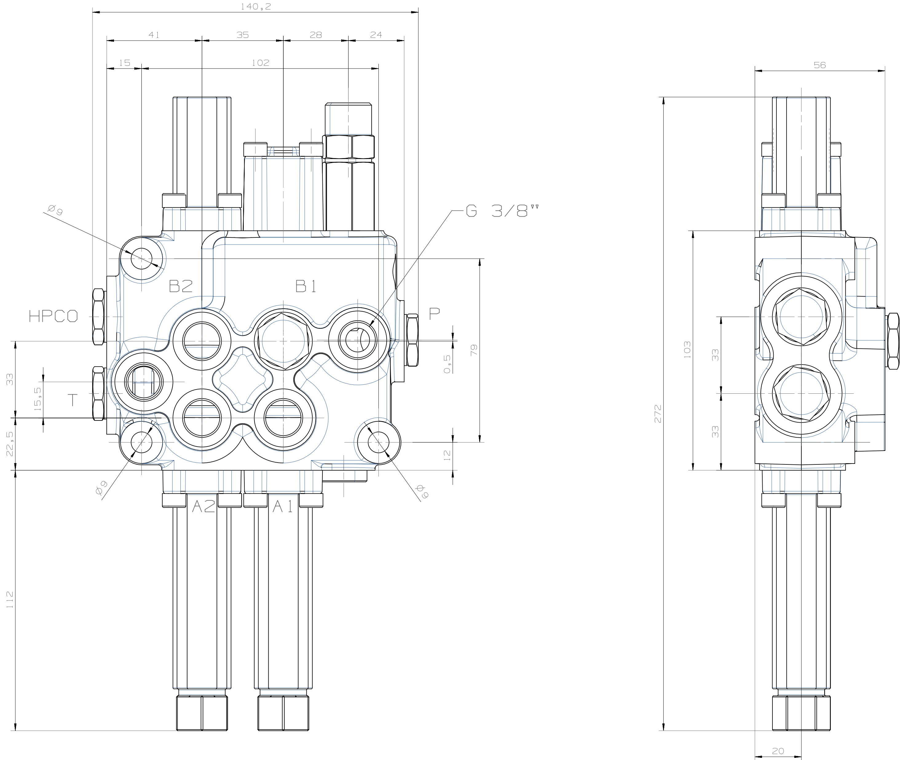
2D-Zeichnung
