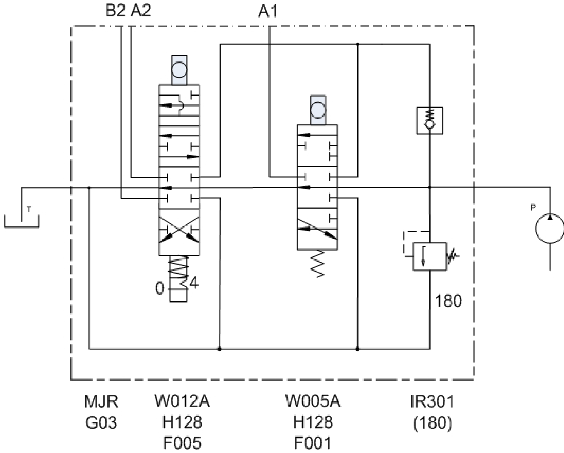
Hydraulikschema
